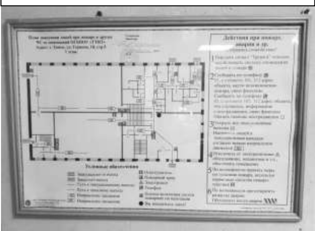
Фото 79 – План эвакуации I этаж
